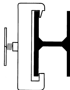
Morsetto tipo A: a doppio bloccaggio e a serraggio a vite
