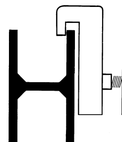
Morsetto tipo B: a bloccaggio singolo e a serraggio a vite
